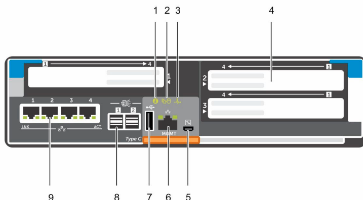
Figure 5. Contrôleur de stockage SC7020
