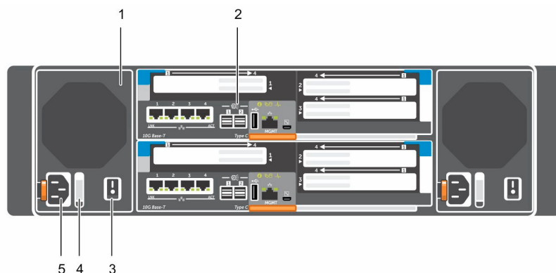
Figure 2. Vue du panneau arrière du Système de stockage SC7020
